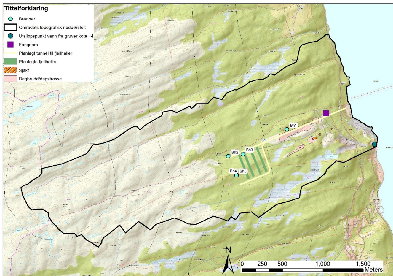
Figur 1: Fjellhallene er planlagt vest for dagens nedlagte gruver og deponier. Brønnene Bh1-Bh5 er etablert for å gi informasjon om hydrogeologiske og geologiske forhold i berget [4]. På kote +4 er det et utløp for vann fra nedlagte gruver. Sorte koter i kartet er koter for mengde naturlig overflateavrenning [7].
