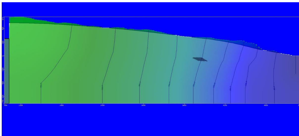
Figur 14: Grunnvannsspeilet er markert med en mørk strek under terrengoverflaten. Fjellhallen ligger i området markert med en mørkere farge (diamant).
