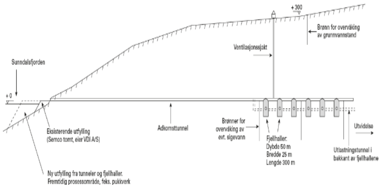
Figur 2: Grov prinsippskisse av planlagte fjellhaller med adkomsttunnel [8].
