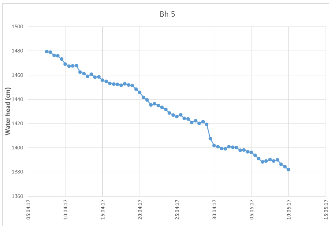
Figur 7: Grunnvannsnivåer i brønn Bh5 logget med Diver fra 7.april 2017 til 10. mai 2017
