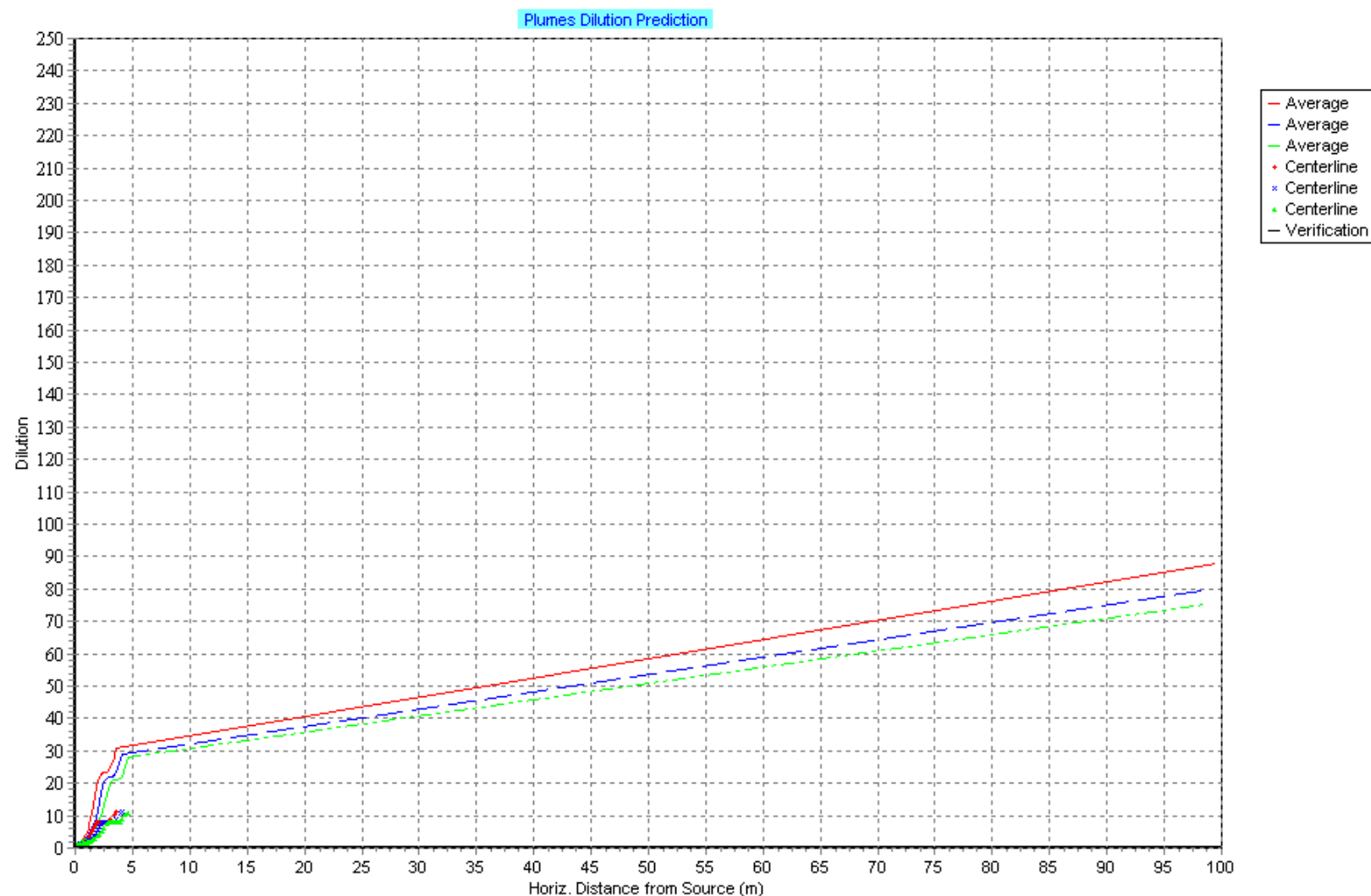
Figur 37: Utslippet fortynning i resipienten med rent sjøvann. Sommer, rørdiameter: 30 cm, utslippsdyb 15 m. Rød 300 000 m³/år, blå 400 000 m³/år og grønn 500 000 m³/år. Linje viser gjennomsnitt av utslippet, prikker viser senterlinjen.
