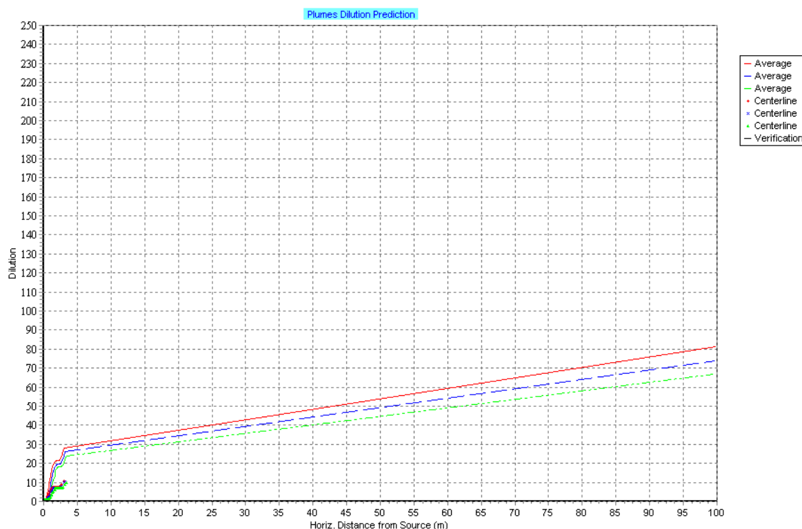
Figur 10: Utslippet fortynning i resipienten. Sommer, rørdiameter: 45 cm, utslippsdyp 15 m. Rød 300 000 m 3 /år, blå 400 000 m 3 /år og grønn 500 000 m 3 /år. Linje viser gjennomsnitt av utslippet, prikker viser senterlinjen.
