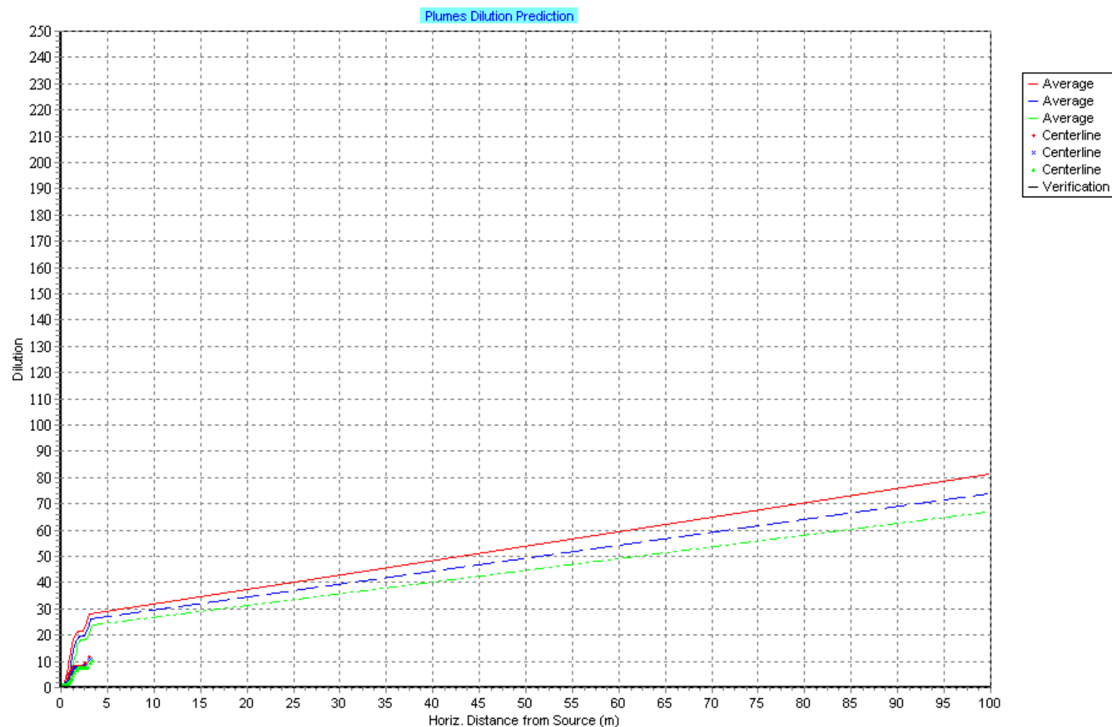
Figur 48: Utslippet fortynning i resipienten med rent sjøvann. Sommer, rørdiameter: 45 cm, utslippsdyb 15 m. Rød 300 000 m³/år, blå 400 000 m³/år og grønn 500 000 m³/år. Linje viser gjennomsnitt av utslippet, prikker viser senterlinjen. Med konsentrasjon av kadmium i resipient og utslipp. NB: Kun «centerline»-beregninger tar hensyn til konsentrasjon i resipienten.
