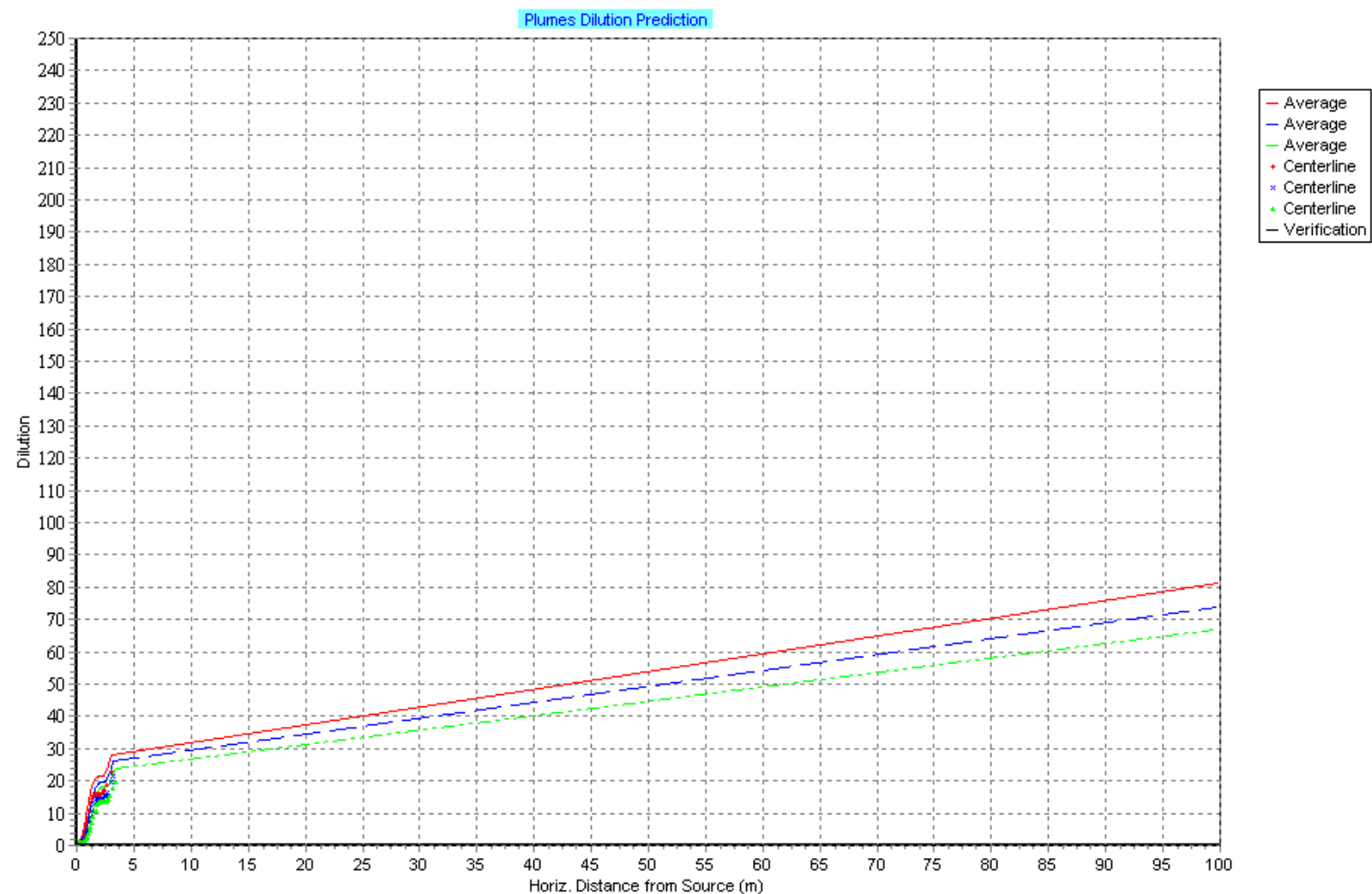
Figur 47: Utslippet fortynning i resipienten med rent sjøvann. Sommer, rørdiameter: 45 cm, utslippsdyp 15 m. Rød 300 000 m³/år, blå 400 000 m³/år og grønn 500 000 m³/år. Linje viser gjennomsnitt av utslippet, prikker viser senterlinjen. Med konsentrasjon av arsen i resipient og utslipp. NB: Kun «centerline»-beregninger tar hensyn til konsentrasjon i resipienten.
