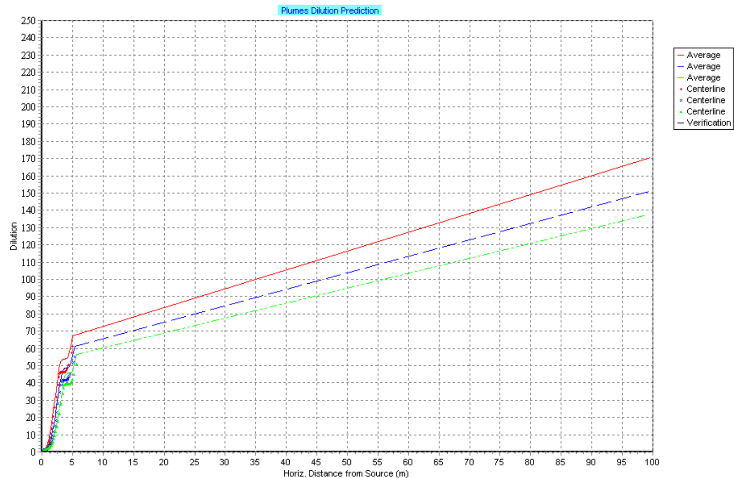
Figur 45: Utslippet fortynning i resipienten med rent sjøvann. Sommer, rørdiameter: 30 cm, utslippsdyp 30 m. Rød 300 000 m³/år, blå 400 000 m³/år og grønn 500 000 m³/år. Linje viser gjennomsnitt av utslippet, prikker viser senterlinjen. Med konsentrasjon av arsen i resipient og utslipp. NB: Kun «centerline»-beregninger tar hensyn til konsentrasjon i resipienten.
