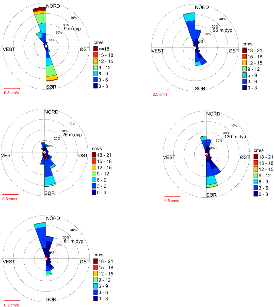
Figur 13. Strømroser av modellert strøm fra dumpeområdet for perioden september – oktober 2014. Totallengden på sektorene indikerer andel målinger (%) i respektive retninger i løpet av måleperioden. Lengden på hvert fargesegment i hver sektor bestemmer videre den relative andelen av målinger med korresponderende strømstyrke (se fargeskala) innenfor hver enkelt sektor. For eksempel, jo mer gul farge i en sektor, desto mer strøm med styrke 12 – 15 cm/s i den sektoren. Rød pil indikerer størrelse og retning på middelstrømmen. Skaleringspil (0.5 cm/s mot øst) er vist i nede til venstre i hver figur.
