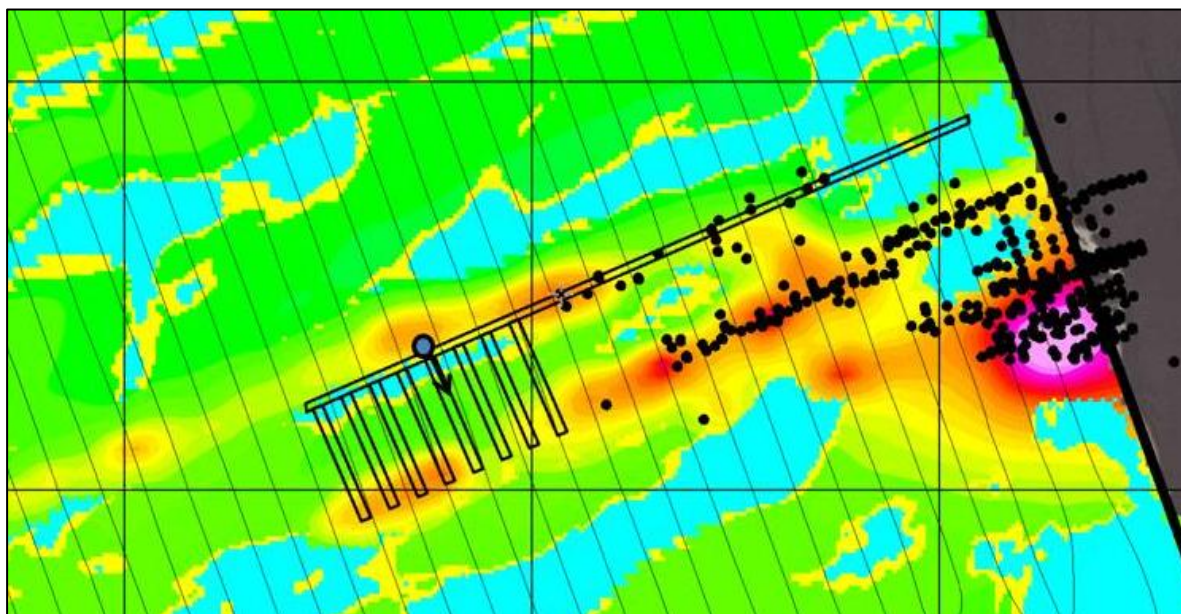
Figur 9: Magnetisk totalfelt (grønt - gult - rødt) overlagret dypforvittringsanalyse (blått med gult omriss) ved Raudsand. Anbefalt boring angitt med sirkel (standplass) og pil for boreretning.
