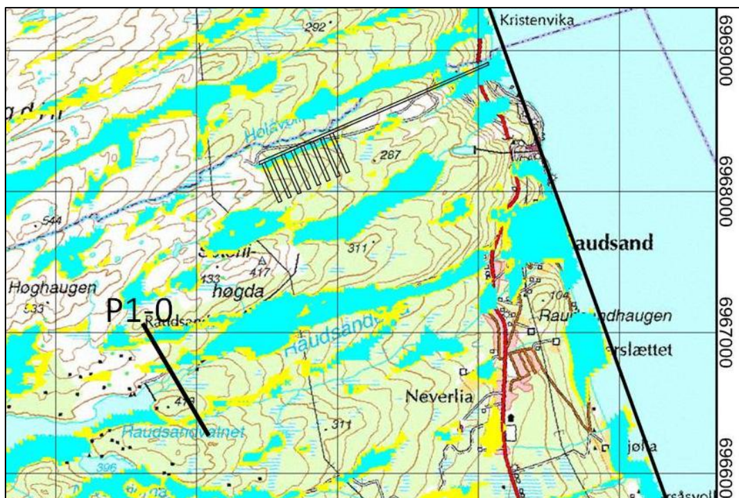
Figur 7: Lokalisering av tidligere resistivitetsprofil for kartlegging av svakhetssone ved Raudsand (fra Nasuti et al. 2009).
