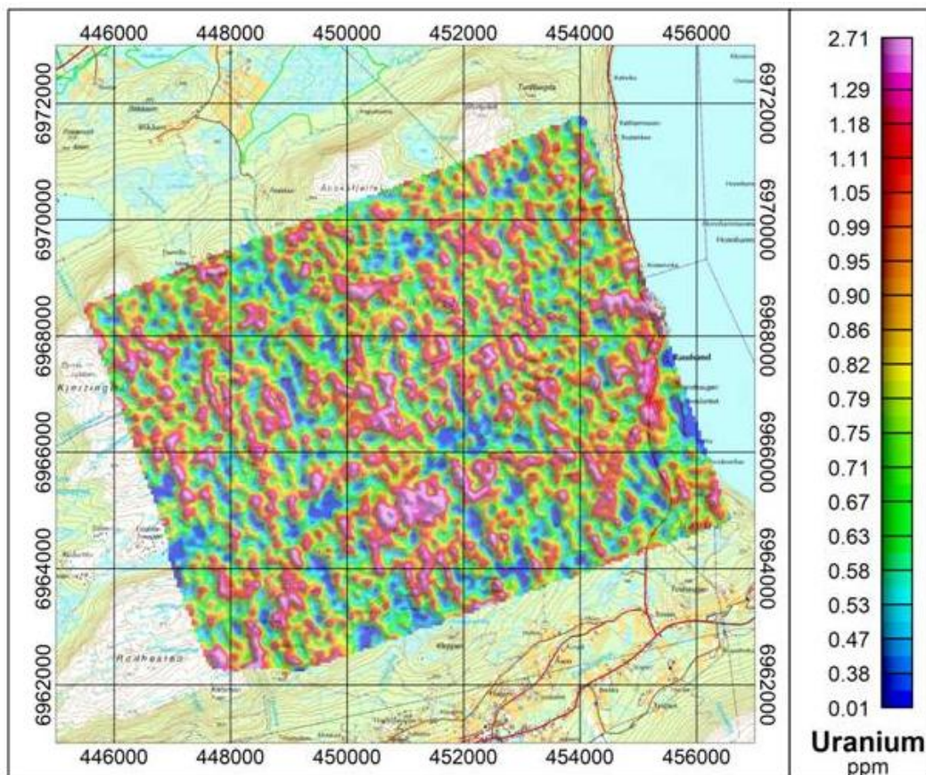
Figur 11: Målt konsentrasjon av uran på bakken.
